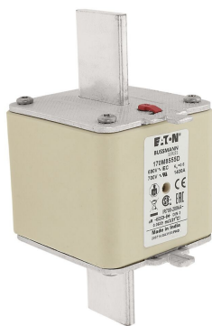
170M8555D
