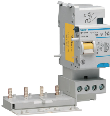
BF425N
