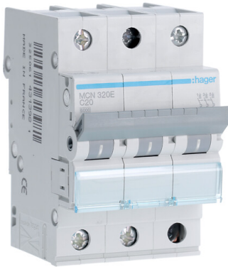
MCN320E
